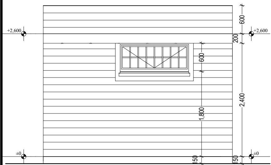
ELEVATION 01
