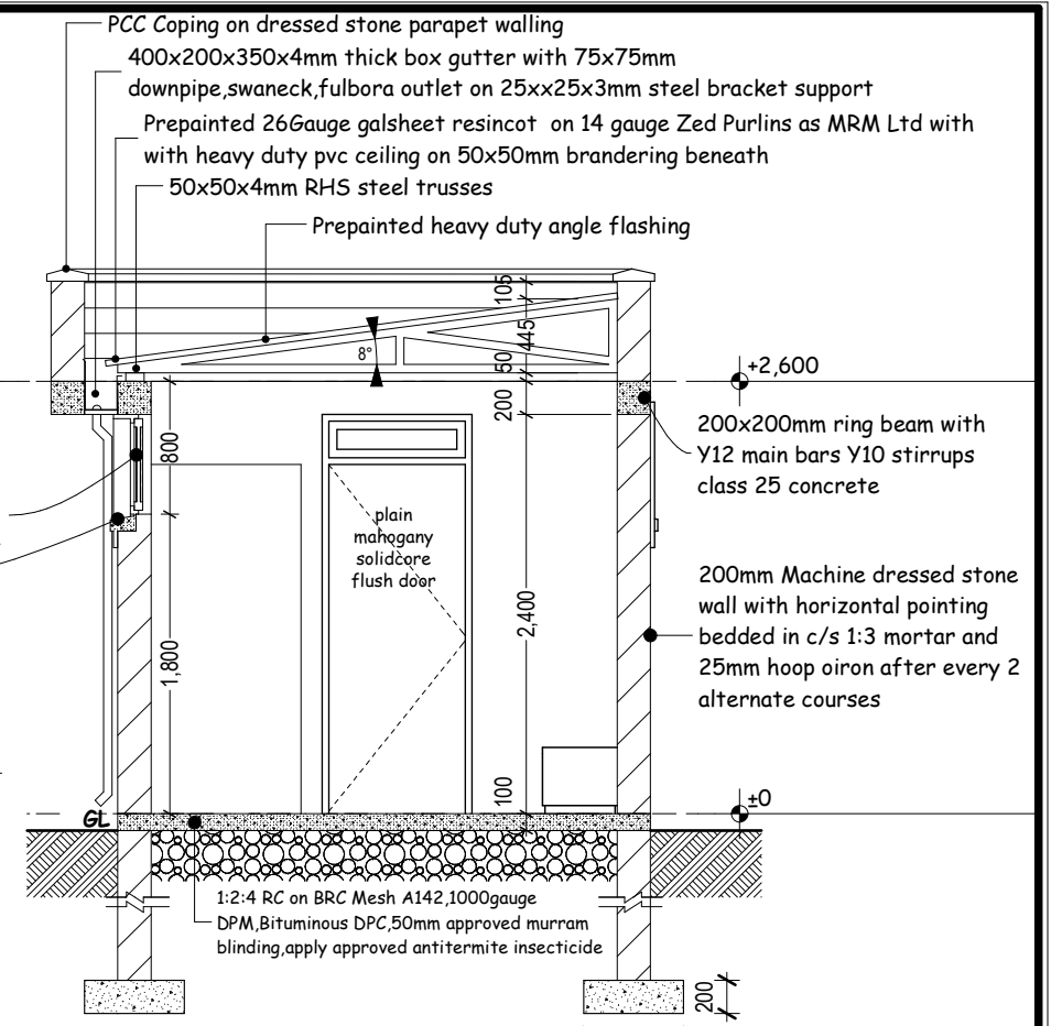
SECTION A-A
