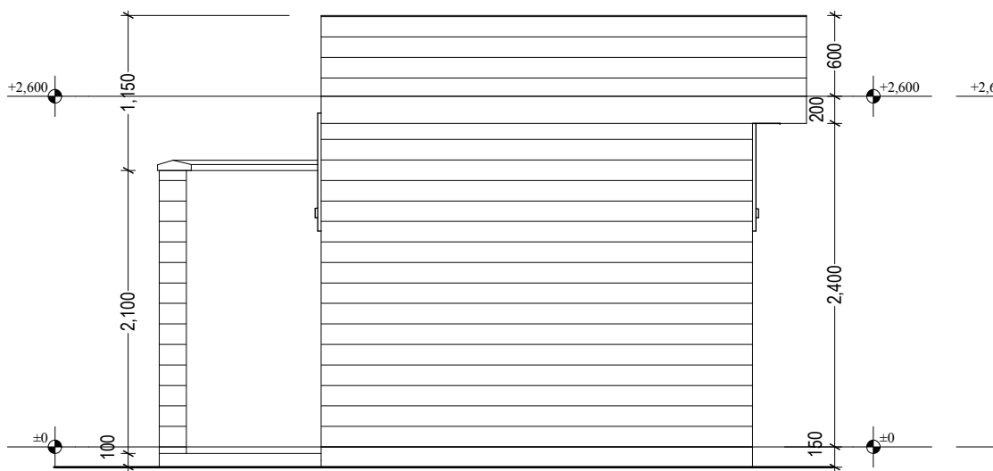
ELEVATION 02
